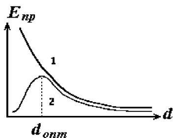
Рис. 1.32. Зависимость электрической прочности слоистых диэлектриков от толщины
