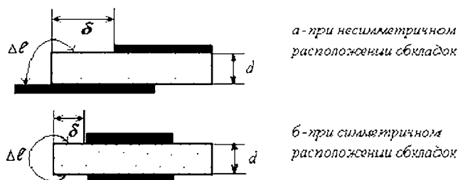
Рис.2.1. Схема расположения обкладок
