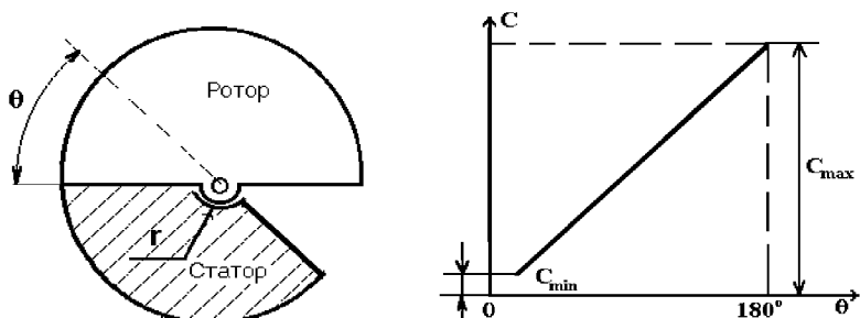
Рис.3.2. Прямоемкостной конденсатор
