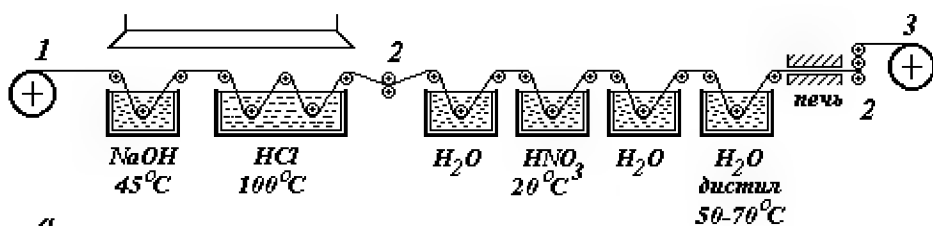
Химический метод динамического травления
