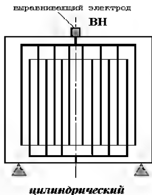
Рис. 3.6. Конструкции газонаполненных конденсаторов
