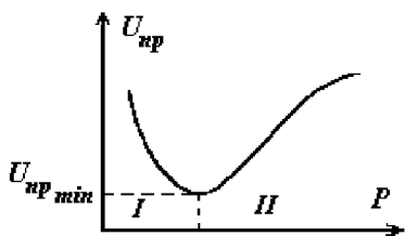
Рис.1.30. Зависимость пробивного напряжения газа от давления
