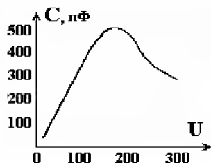
Рис.3.17. Зависимость C=f(U) для варикондов ВК1
