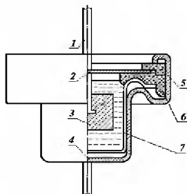
Рис.3.34. Танталовый электролитический конденсатор с объемно-пористым анодом: 1- вывод, 2 – крышка, 3 – анод, 5 – уплотнение, 6 – изоляционная прокладка, 7 – металлический корпус
