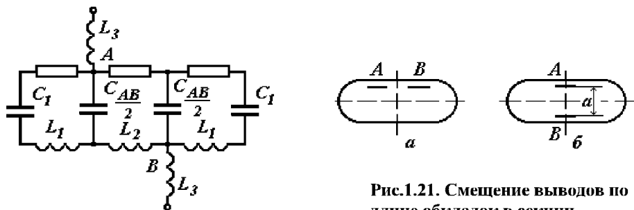
Рис.1.20. Эквивалентная схема замещения секции со смещенными обкладками
