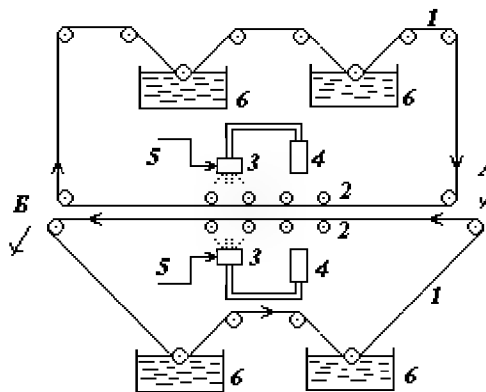
Рис. 3.12 Схема автомата для серебрения слюды методом окисления: 1. Конвейерная лента. 2. Нажимные ролики. 3. Пульверизаторы. 4. Резервуары с пастой. 5. Сжатый воздух. 6. Ванны для очистки конвейерных лент. А-Укладка слюды. Б-Сброс пластин
