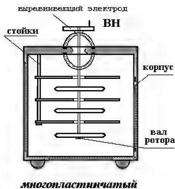
Рис. 3.6. Конструкции газонаполненных конденсаторов
