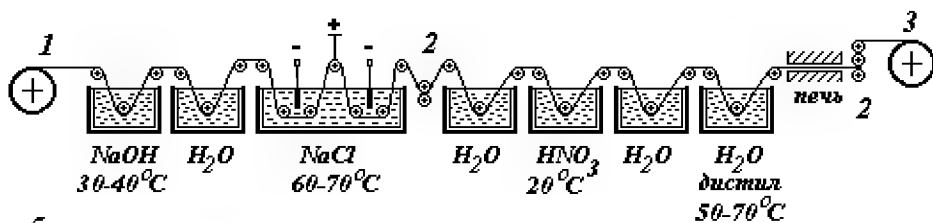
Электрохимический метод динамического травления
