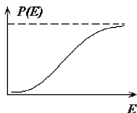
Рис.1.33. Интегральная кривая распределения пробивных напряженностей электрического поля
