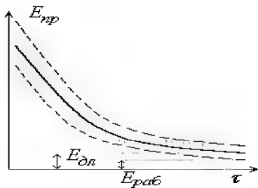
Рис. 1.35. Зависимость электрической прочности от времени старения
