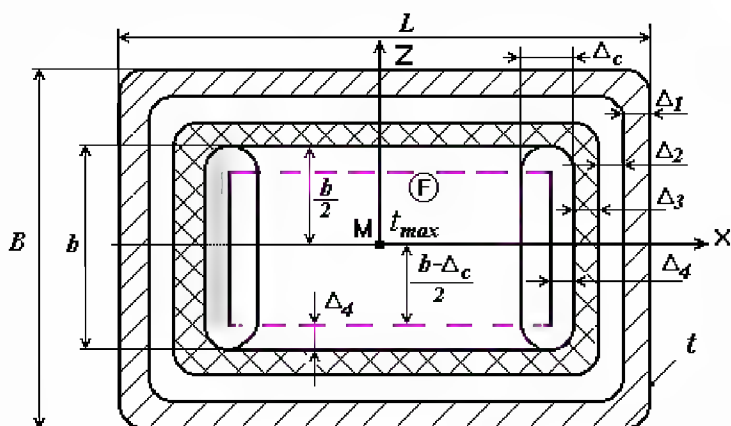
Рис.2.8. Схема распределения температуры внутри конденсатора
