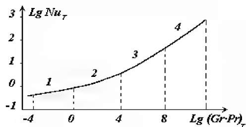
Рис. 2.4. Зависимость Lg Nu от Lg произведения Gr \cdot Pr
