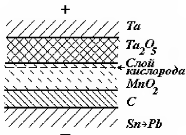
Рис.3.33. Принципиальная схема твердого танталового электролитического конденсатора
