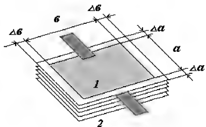
Рис. 3.11. Сечение пластин слюды (2) с напыленными обкладками (1)
