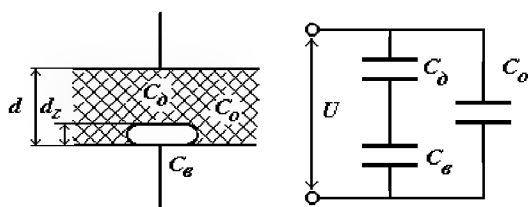
Рис.1.36. Эквивалентная схема замещения диэлектрика с воздушным включением:
