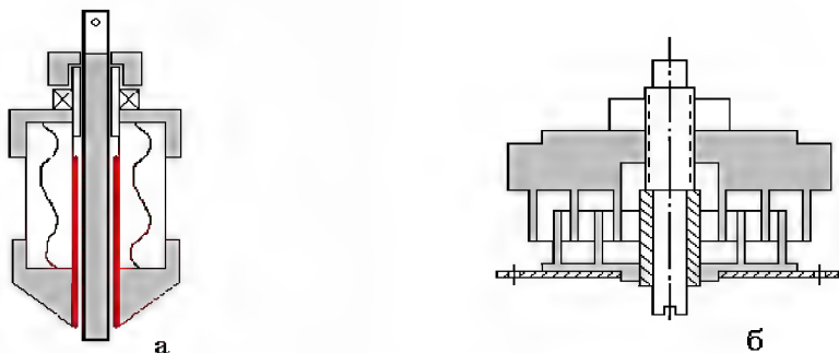
Рис. 3.4. Подстроечные воздушные конденсаторы а) цилиндрические; б) многопластинчатые
