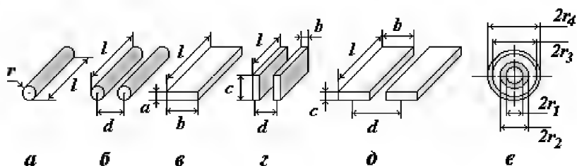
Рис.1.22. Типы проводников в конденсаторах
