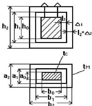
Рис.2.7. Схема расположения секций конденсатора в корпусе
