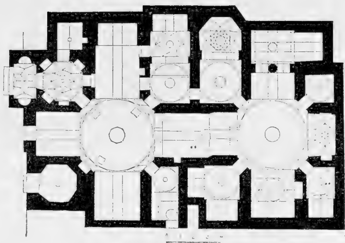
64. Баня Гаджи-хаммам в Баку. План
