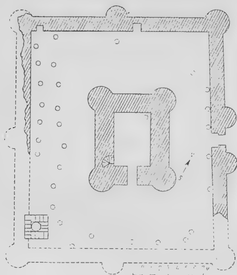
21. Башня-замок в селении Мардакяны. План
