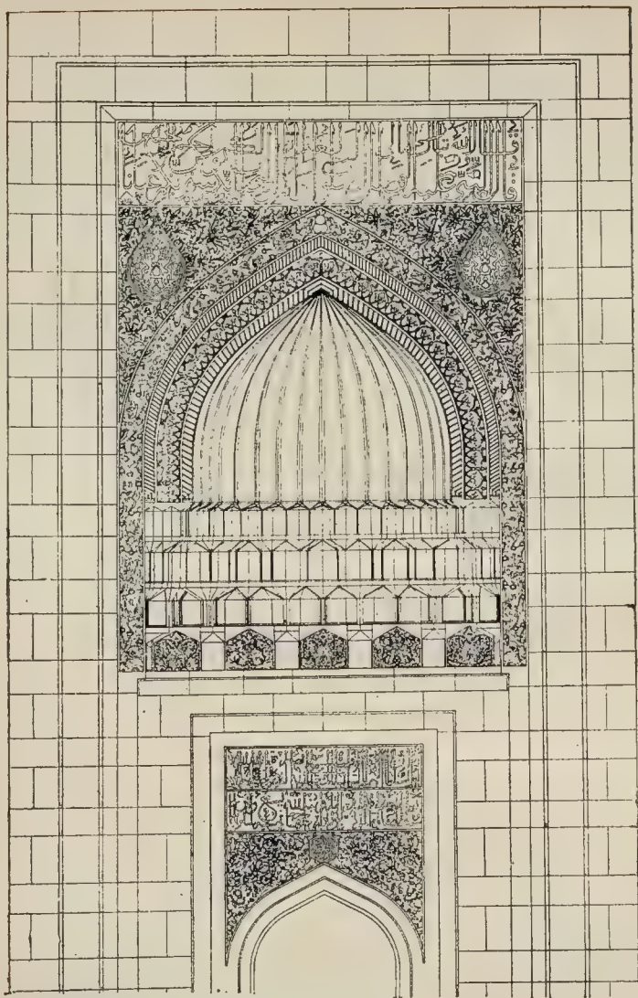
34. Тюрбе. Разрез по продольной оси
