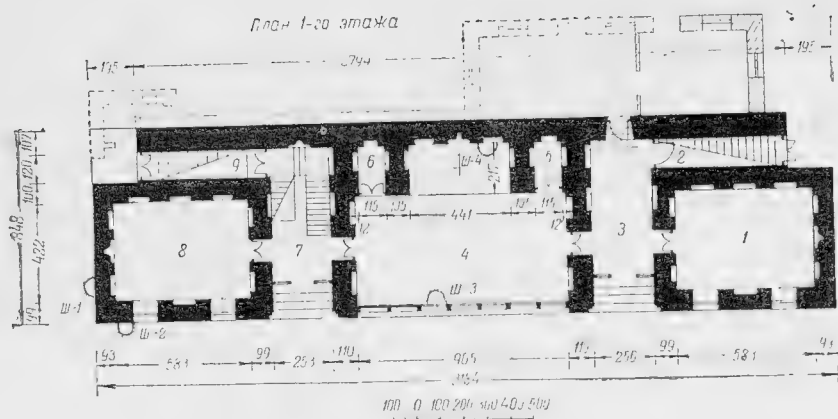
56. Нухинский дворец. План 1 этажа
