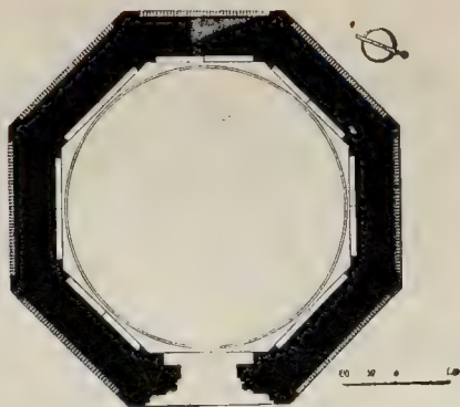
2. Мавзолей Юсиф-ибн-Кусайира в Нахичевани. План
