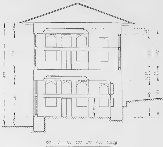
57. Нухинский дворец. Разрез
