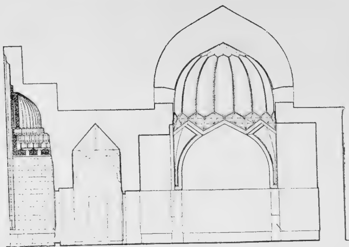
35. Тюрбе. Портал и входной проем
