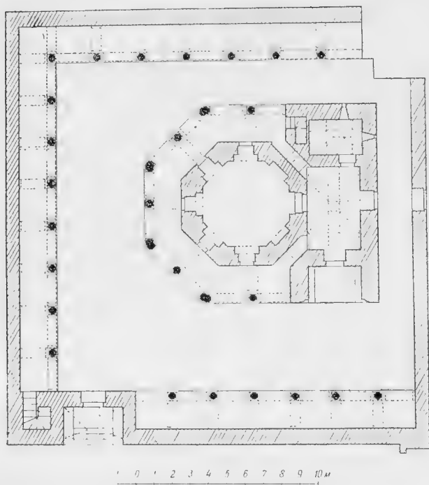
40. Диван-хане. План
