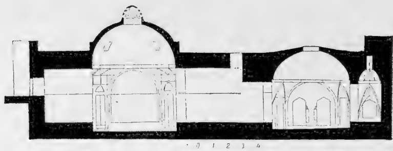
65. Баня Гаджи-хамам в Баку. Разрез
