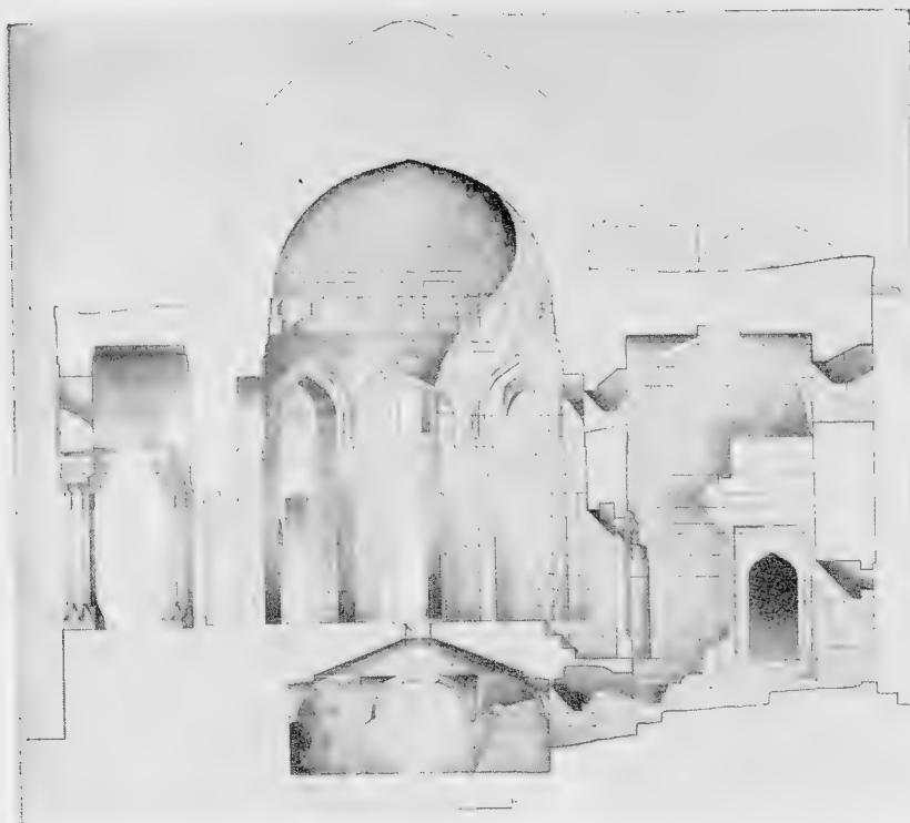
41. Диван-хане. Разрез
